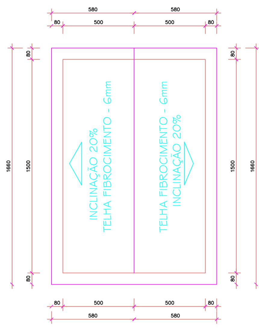
COBERTURA Escala 1/125
