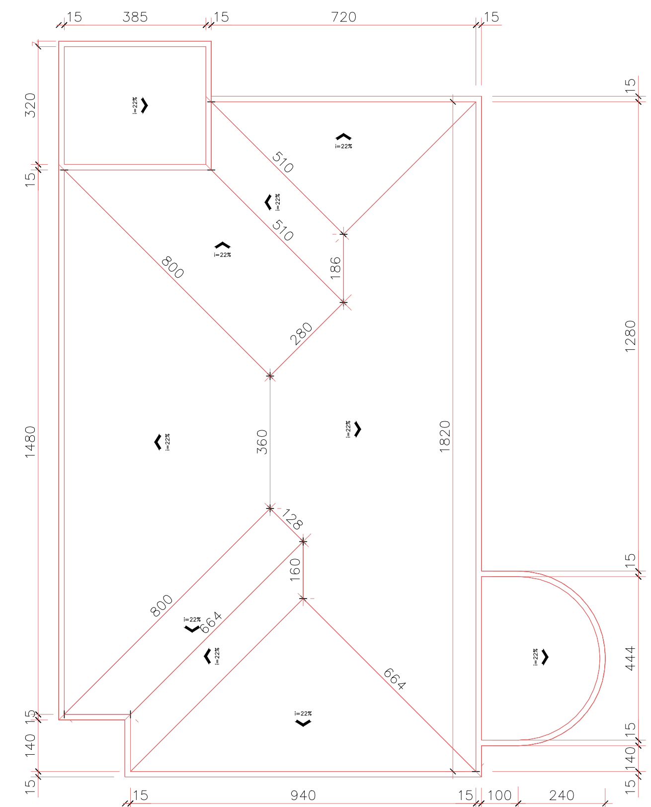
PLANTA DE COBERTURA ESC: 1/100
