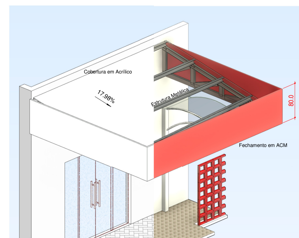
2 Detalhe Alpendre
