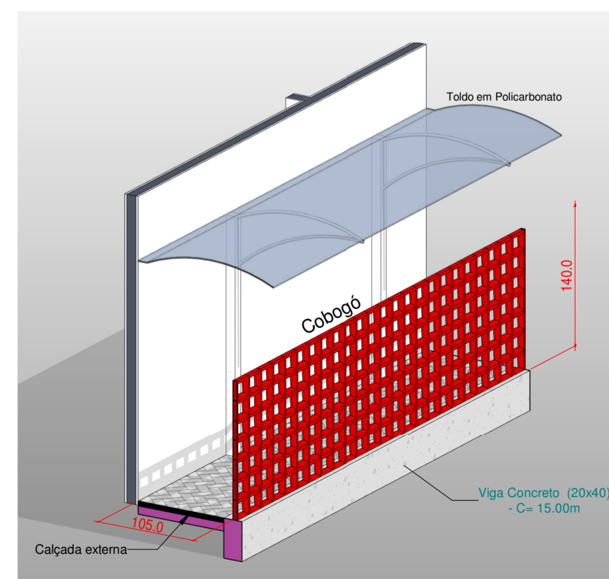
4 Detalhe Toldo
