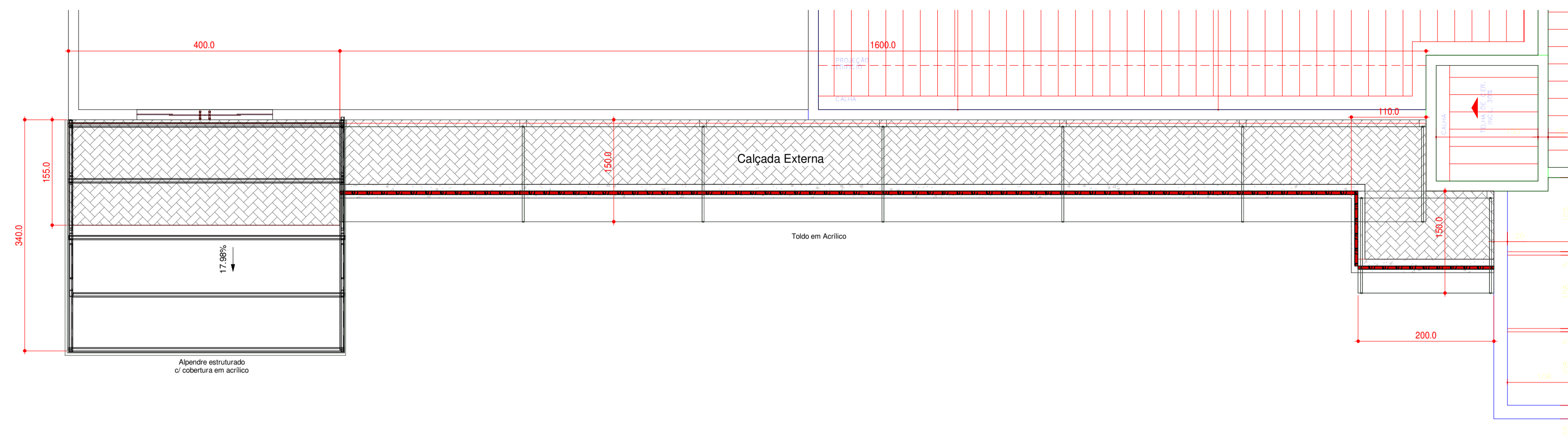
1 Piso Térreo 1 : 50
