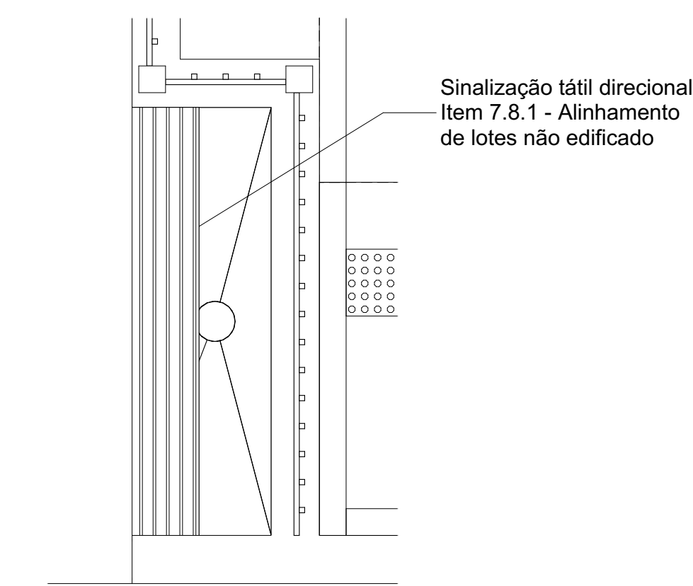
DET06 - Lixeiras 1:20
