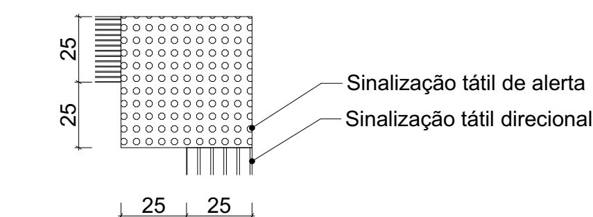
DET07 - Mudança de Direção 90° NBR 16537:2016 / Esc 1:20
