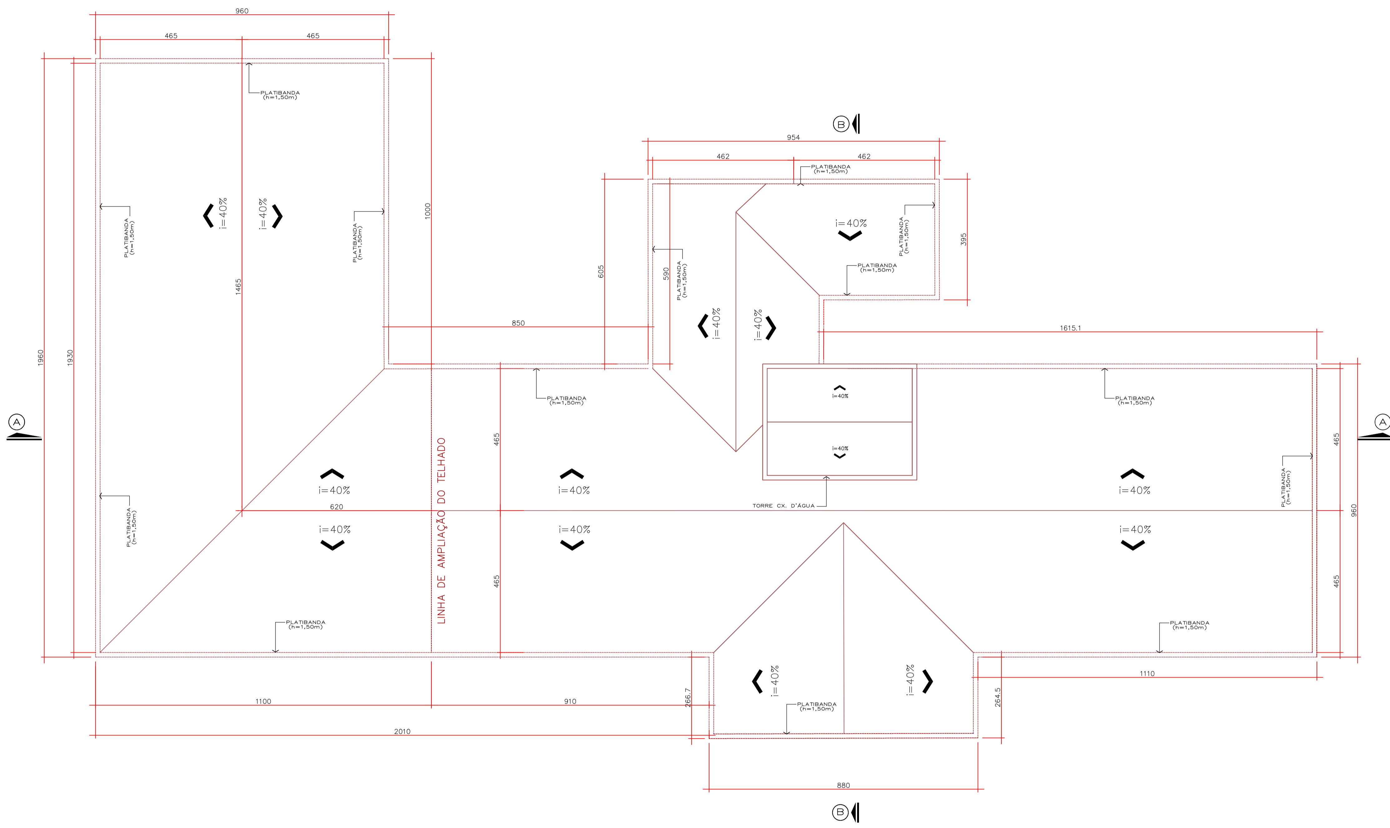
PLANTA COBERTURA ESC = 1/75
