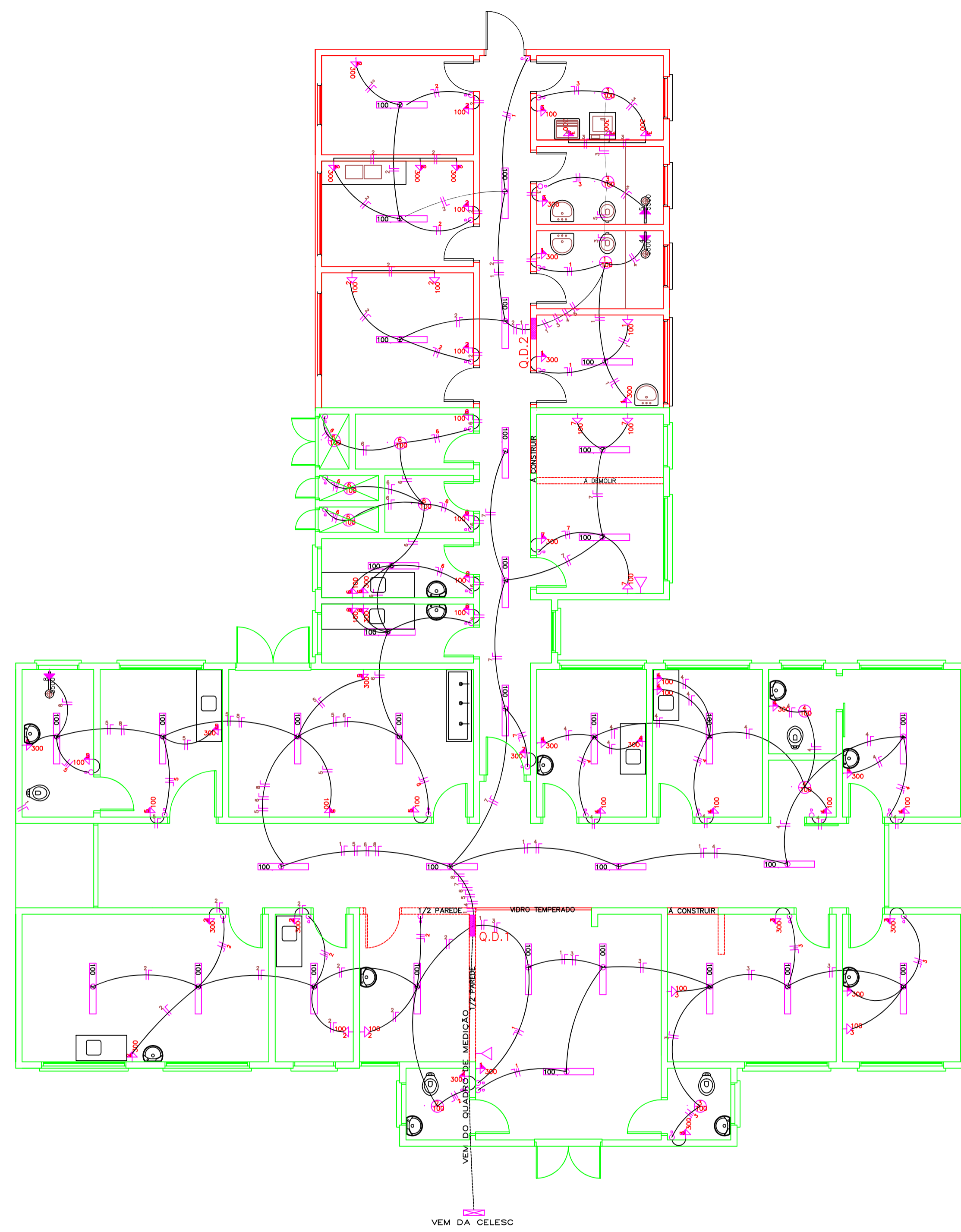
PLANTA BAIXA ELÉTRICO ESC=1/75
