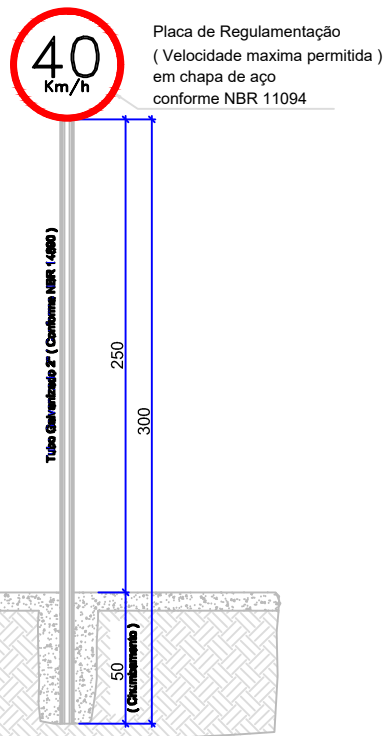
DETALHE ESQUEMATICO ESC: 1/15 CONFORME NBR 14932
