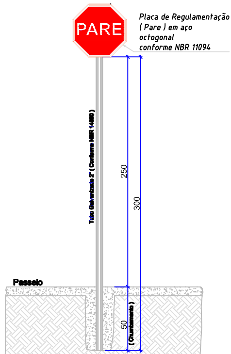
DETALHE ESQUEMATICO ESC: 1/15 CONFORME NBR 14932
