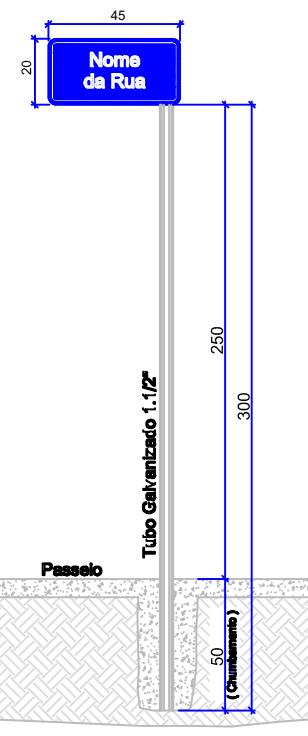
DETALHE ESQUEMATICO ESC: 1/15 PLACA COM O NOME DA RUA
