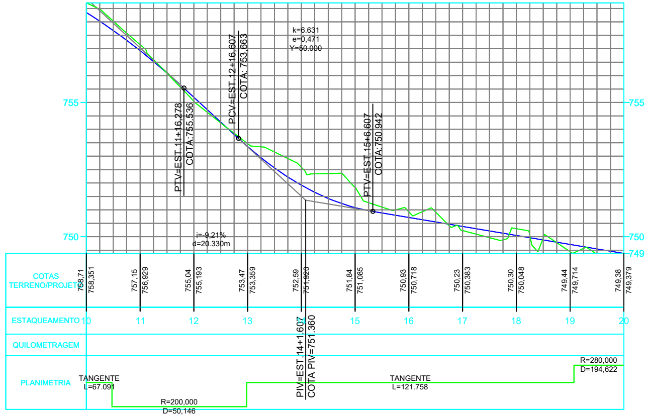
PERFIL LONGITUDINAL RODOVIA LINHA SÃO SEBASTIÃO
