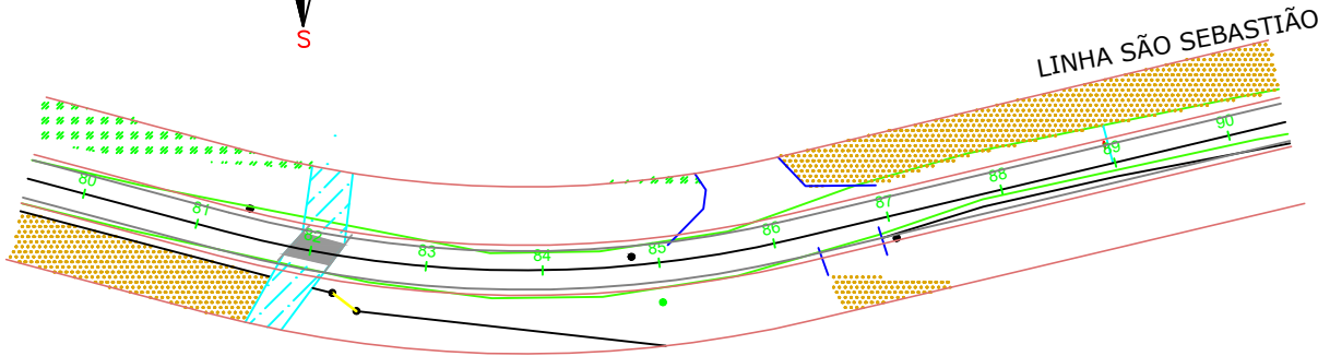
ESTAQUEAMENTO ESC HOR. 1/1000
