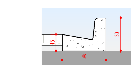
3 Sarjeta 1:20
