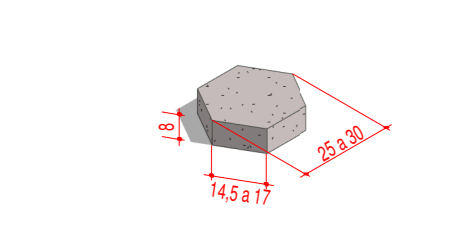
4 Detalhe Lajota
