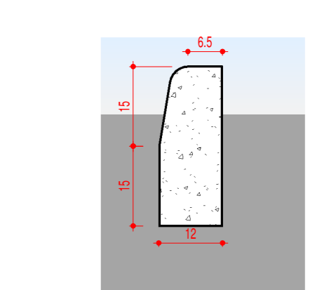
2 MEIO-FIO 1:10
